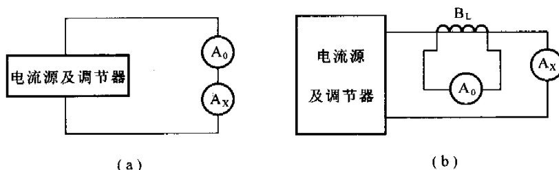
图4 检定电流表的接线图
