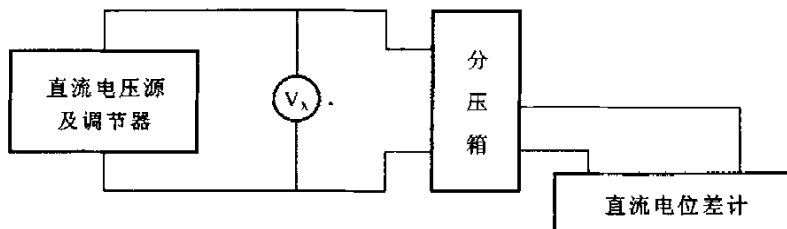
图 9 检定直流电压表的接线图
