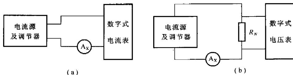
图 1 用数字表检定电流表的接线图
