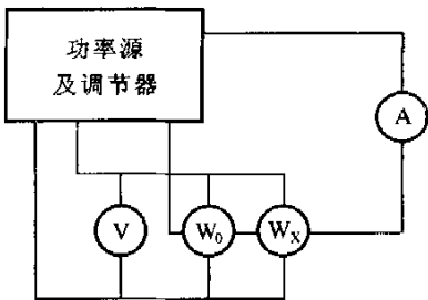
图 6 检定功率表的接线图
