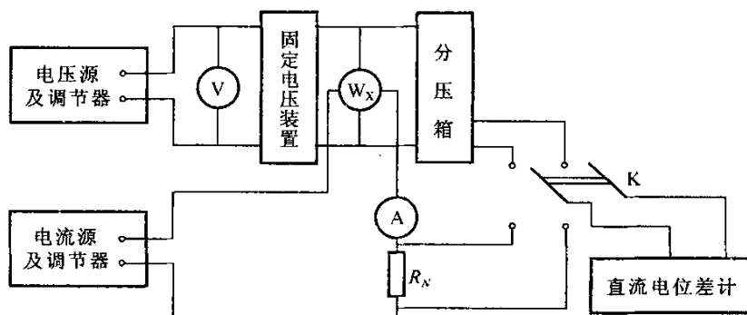
图 10 检定直流功率表的接线图
