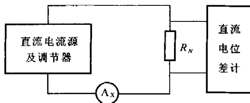
图 7 检定直流电流表的接线图
