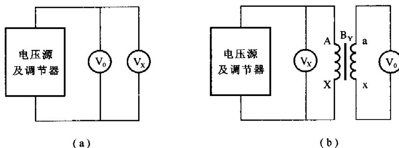
图5 检定电压表接线图
